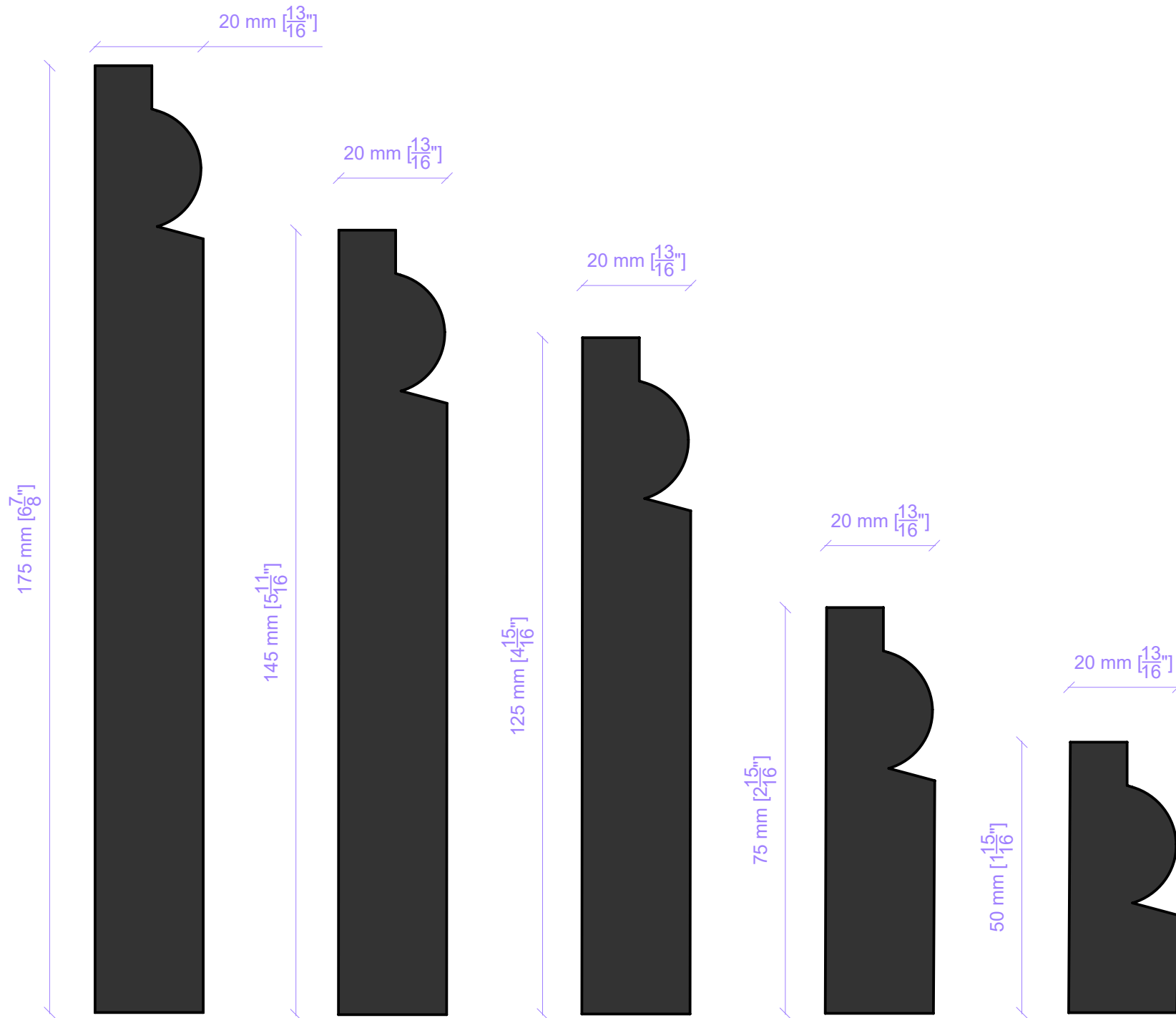
TORUS H MOULDS4
