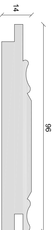
Tongue & Groove 06 1:1 on A4
