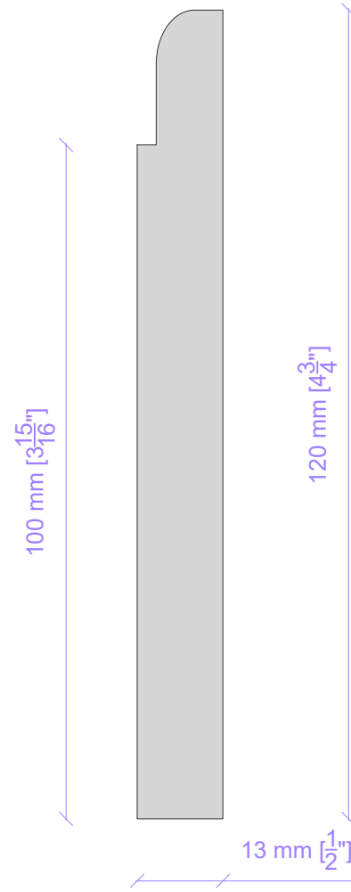
SB10C 1:1 on A4
