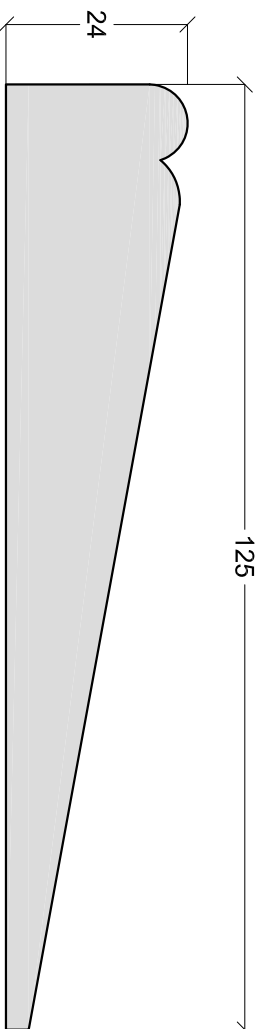
Door Wedge 02 1:1 on A4
