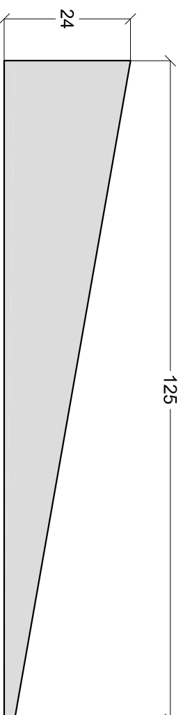
Door Wedge 01 1:1 on A4
