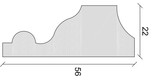
Dado Rail 23 1:1 on A4
