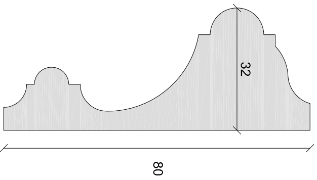
Dado Rail 20 1:1 on A4
