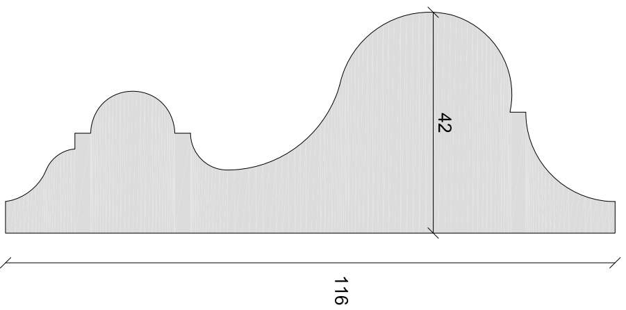
Dado Rail 17 1:1 on A4
