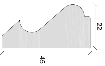
Dado Rail 08 1:1 on A4
