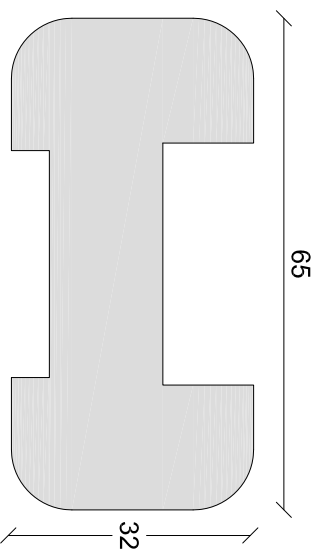
Baserrail 04 1:1 on A4
